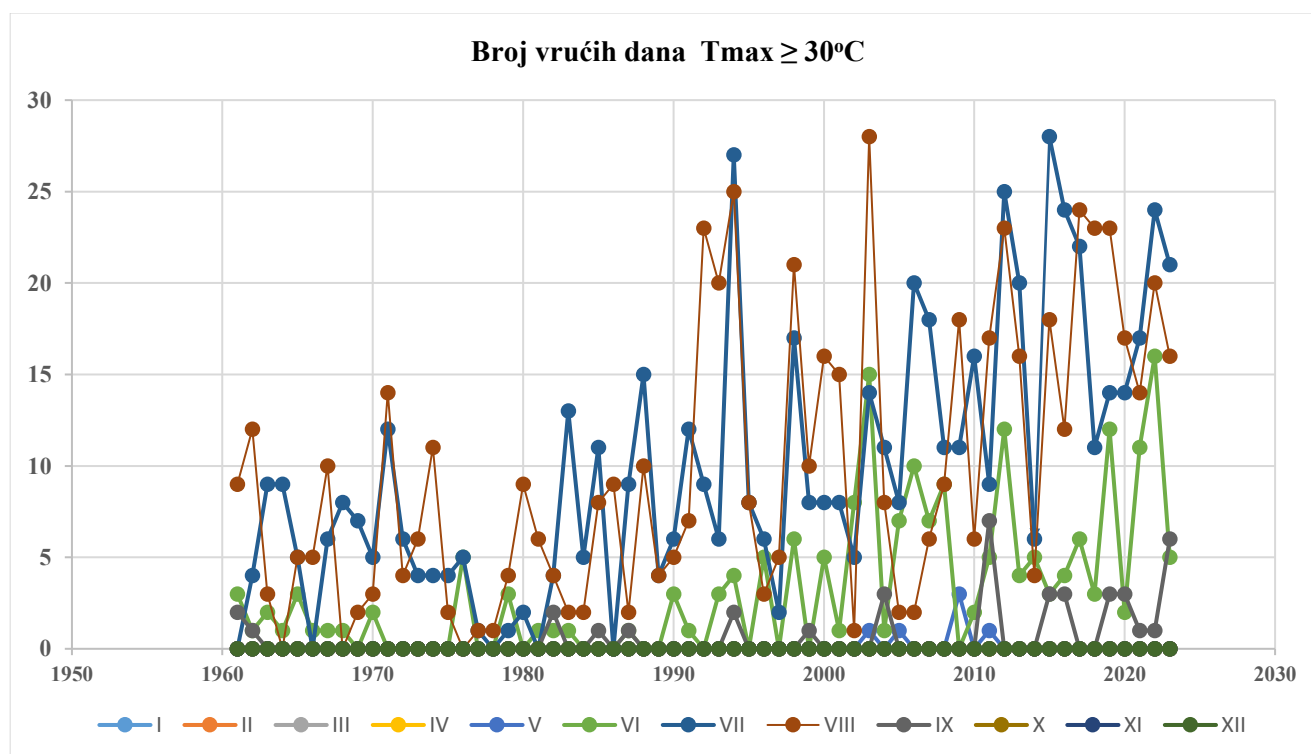
Grafički prikaz 28. Broj vrućih dana T_{max} \geq 30^{\circ}\text{C} .
